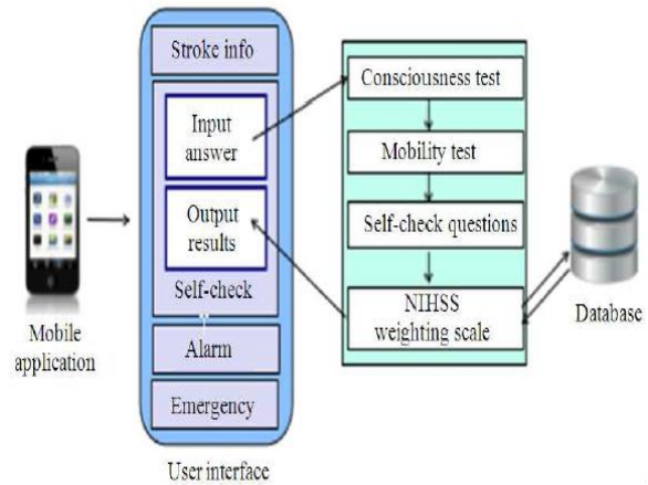
شکل ۲ - معماری پیشنهادشدهی نرم‌افزار Stroke PD برای مدیریت سکته [۷۸]
